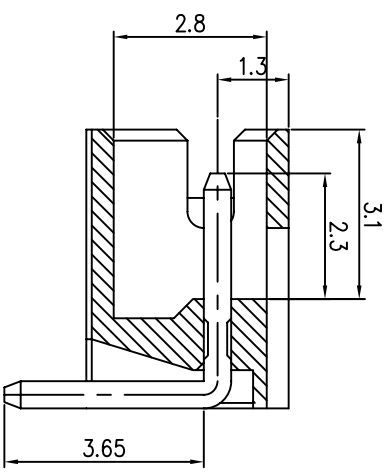
SEC A-A
