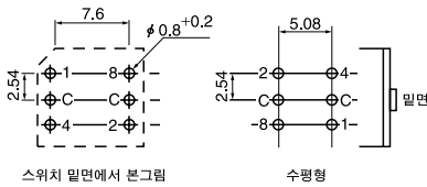
부착 Hole 치수
