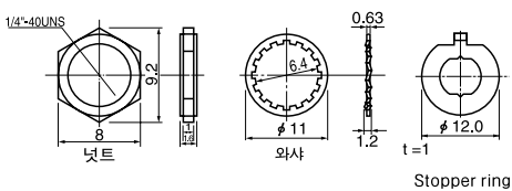
부착 금속구 치수
